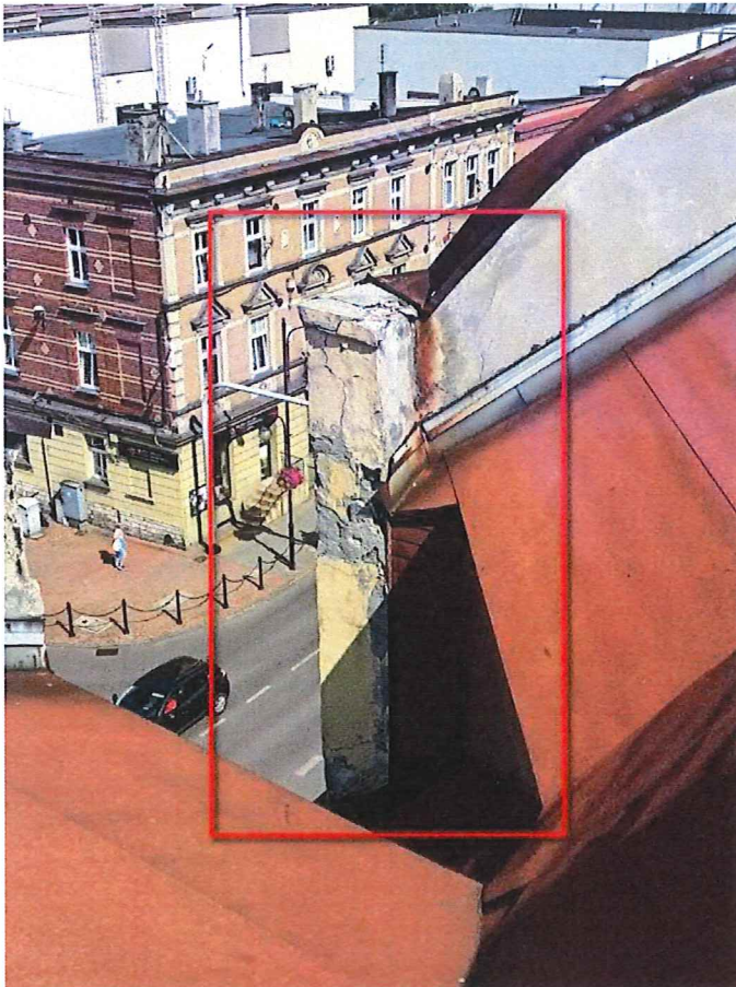
Fot. 7. Zbliżenie na fragment attyki do przemurowania.
