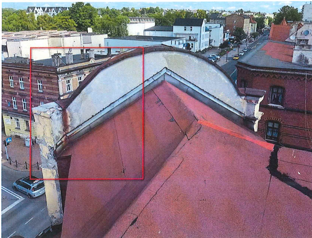
Fot. 8. Zbliżenie na fragment attyki do przemurowania.
