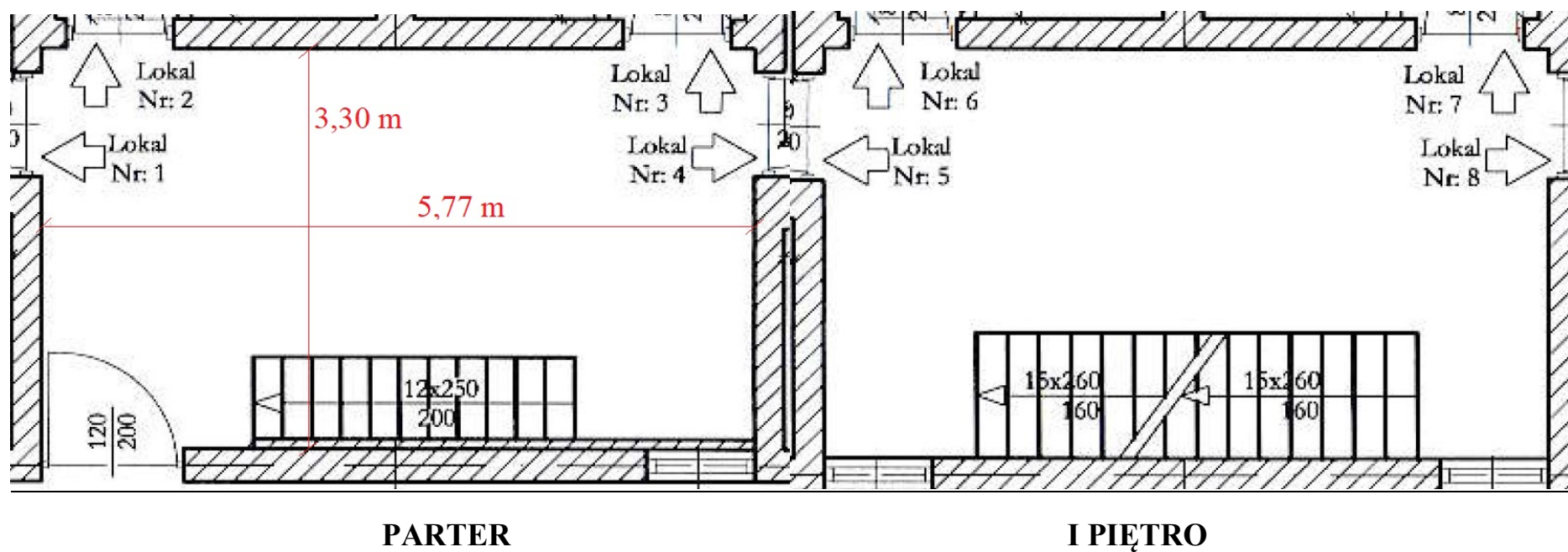
RZUT – KLATKA SCHODOWA Nr I-IV (PARTER – I PIĘTRO klatki schodowe powtarzalne)
