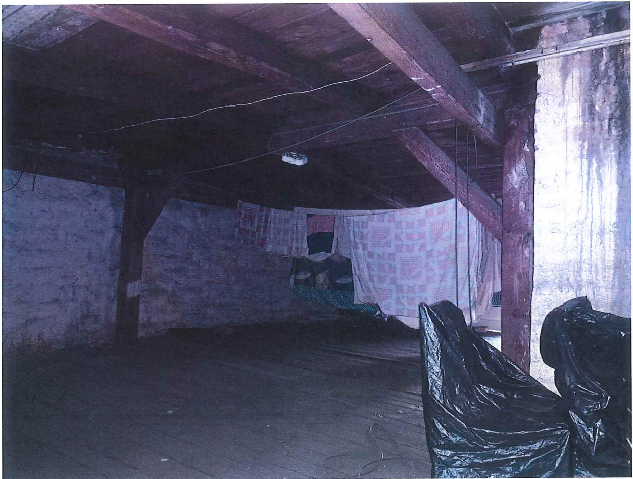
Fot. 13. Widok poddasza nieużytkowanego – więźba dachowa do wzmocnienia lub wykonania na nowo.
