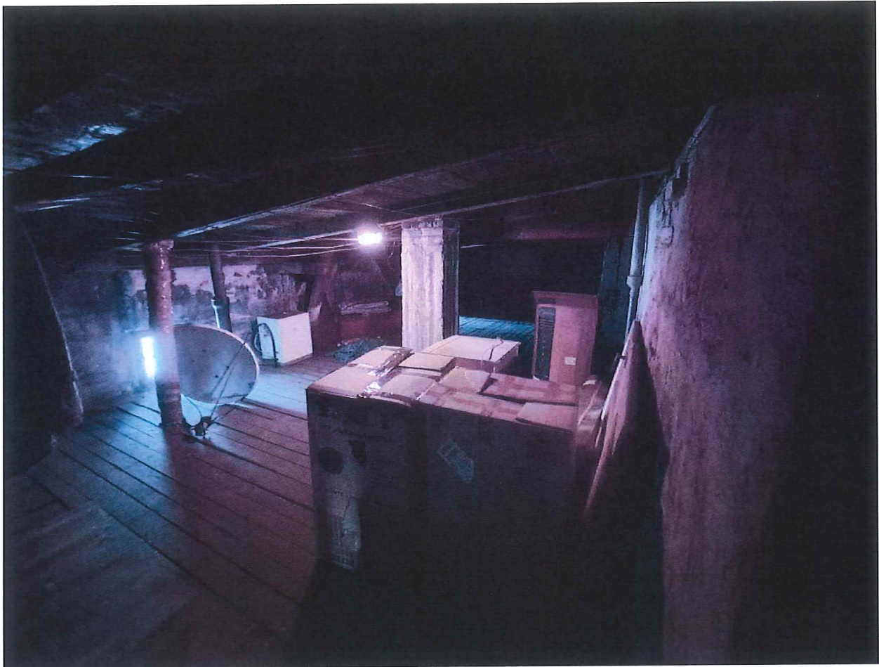
Fot. 10. Widok poddasza nieużytkowanego – więźba dachowa do wzmocnienia lub wykonania na nowo.
