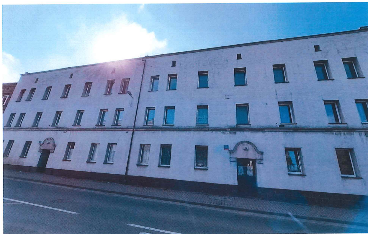
Fot. 2. Widok budynków przy ul. Karola Miarki 15, 16 od frontu.
