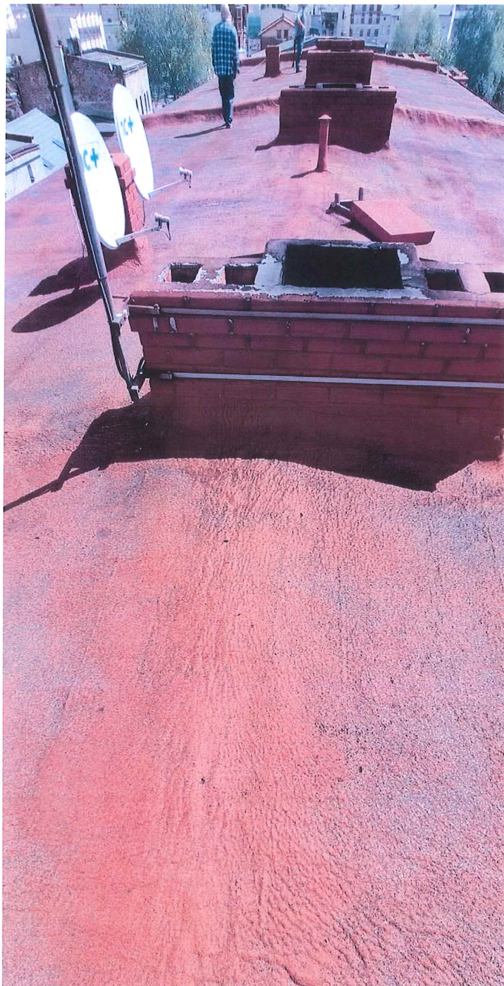
Fot. 4. Widok ogólny połaci dachowej – pianka PUR do usunięcia i utylizacji.
