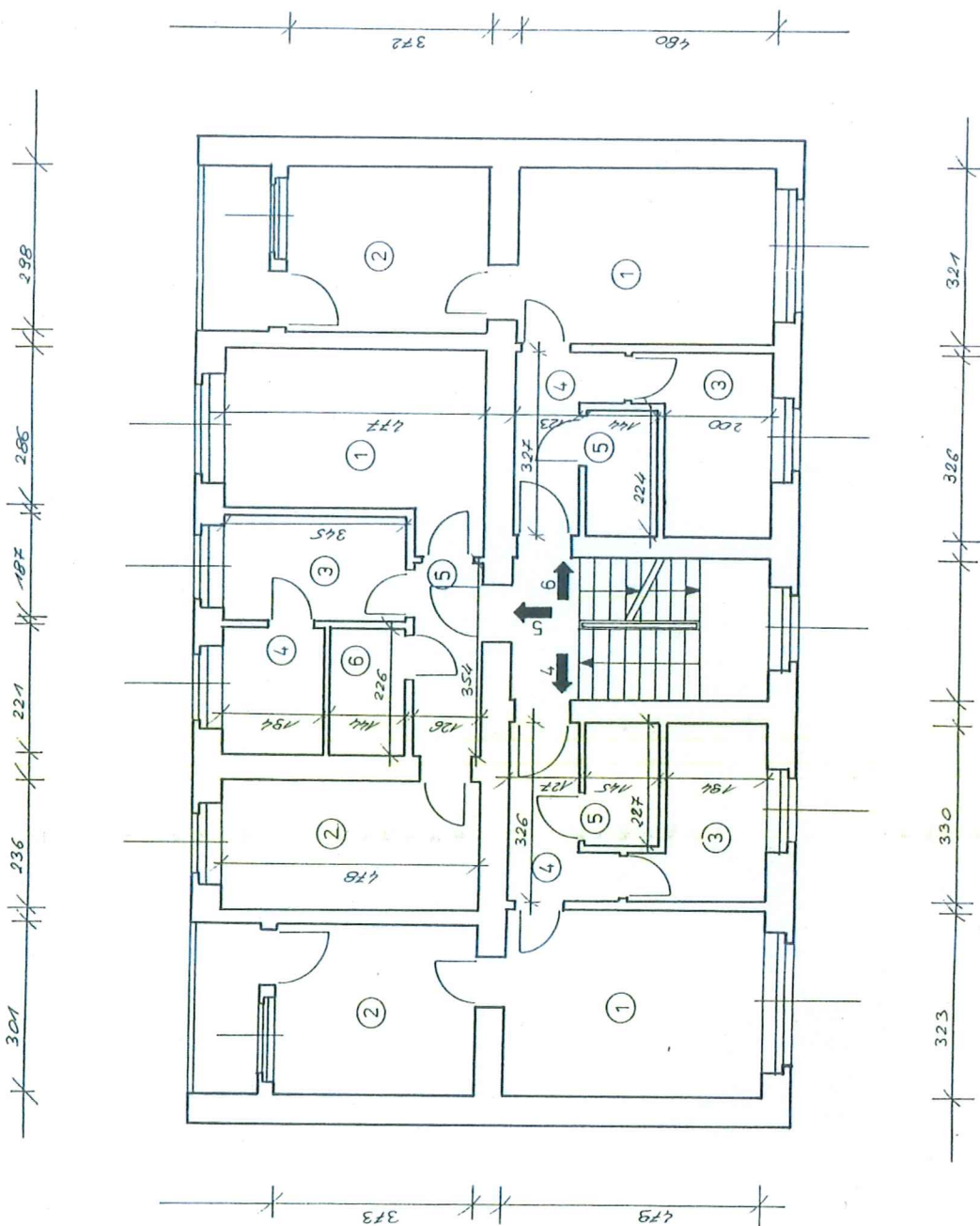
Rzut kondygnacji powtarzalnej – jedna klatka
